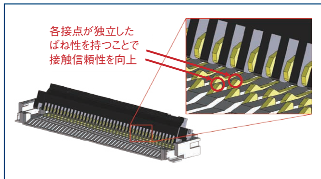
2点接点構造
