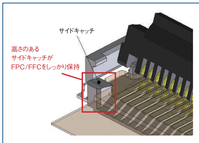
ロック構造による高いFPC/FFC保持力
