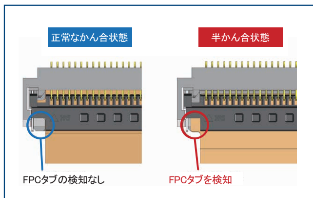
FPC/FFC誤かん合検出
